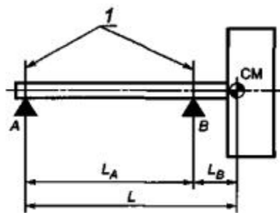
Рисунок 3 - Межопорный ротор с асимметричным расположением центра масс
