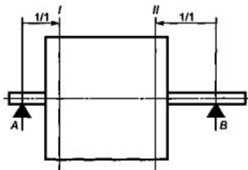
Рисунок Е.1 - Пересчет для плоскостей коррекции, расположенных между плоскостями задания допуска
