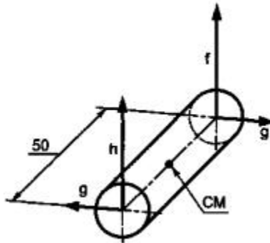
Рисунок 1 - Различные представления одного и того же дисбаланса ротора, лист 1
